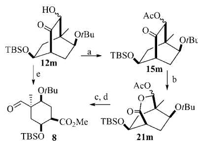
Scheme 6. (a) Ac 2 O, py, DMAP, 0 °C, 1 h 30 min; (b) m -CPBA, NaHCO 3 , CH 2 Cl 2 , 25 °C; (c) K 2 CO 3 , MeOH, 25 °C 1 h 30 min; (d) TMSCHN 2 , Et 2 O, MeOH, 0 °C; (e) Pb(OAc) 4 , toluene, MeOH, 0 °C.
